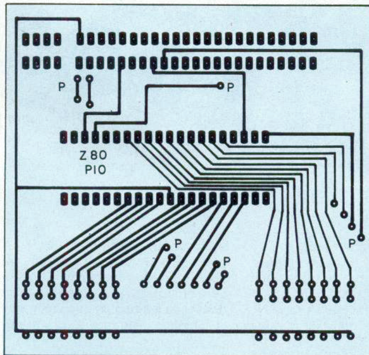
Cara superior de la placa de circuito impreso. Los terminales marcados P corresponden a puentes entre la cara superior y la inferior. En la parte superior de la figura están las pistas del conector al bus de expansión del Spectrum. Las resistencias deben soldarse en las salidas de los dos ports en la parte inferior de la figura.
