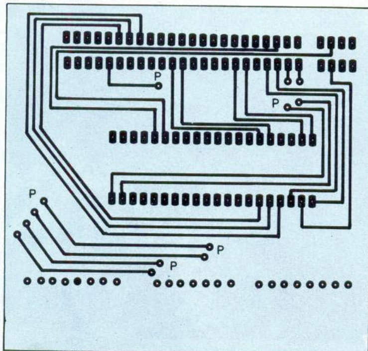
Cara inferior del circuito impreso. Atención a los puentes con la cara superior.
